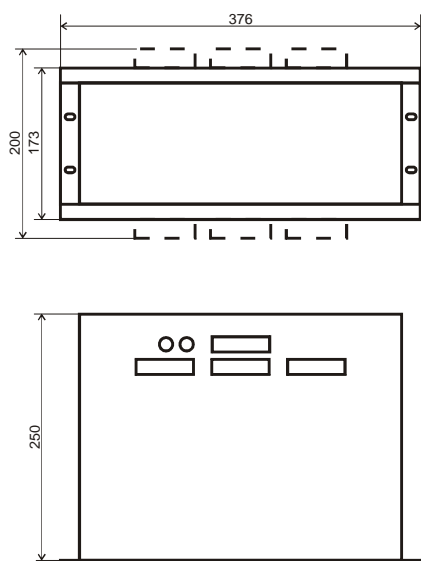
WYMIARY AUTOMATU AZR W WERSJI 10 OBUDOWA ZATABLICOWA KASETA EURO 63T (APRA)
