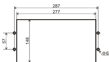
OTWORY W PŁYCE MONTAŻOWEJ
