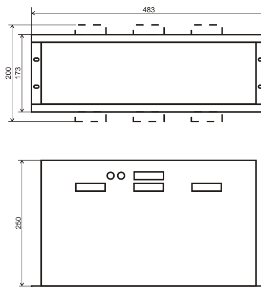
WYMIARY AUTOMATU AZR W WERSJI 11 OBUDOWA ZATABLICOWA KASETA EURO 84T (APRA)
