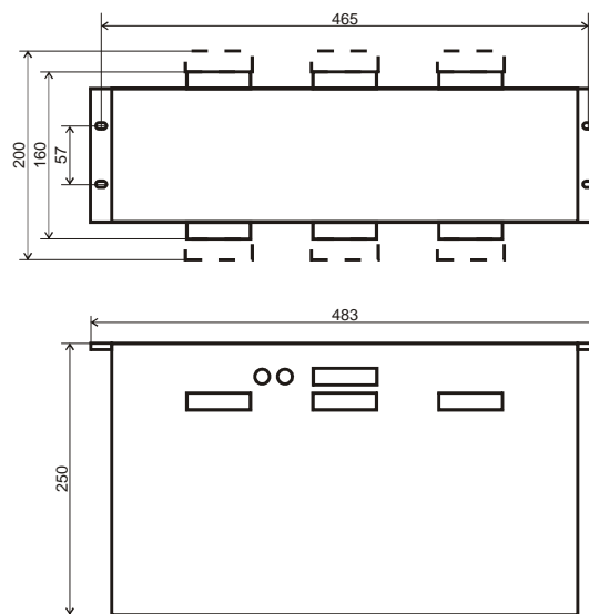
WYMIARY AUTOMATU AZR W WERSJI 9 OBUDOWA NATABLICOWA KASETA EURO 84T (APRA)
