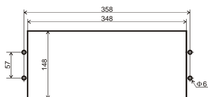
OTWORY W PŁYCE MONTAŻOWEJ
