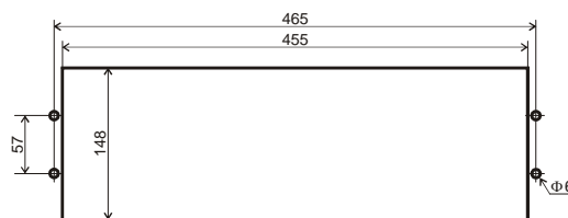
OTWORY W PŁYCE MONTAŻOWEJ
