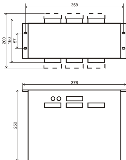
WYMIARY AUTOMATU AZR W WERSJI 5 OBUDOWA NATABLICOWA KASETA EURO 63T (APRA)
